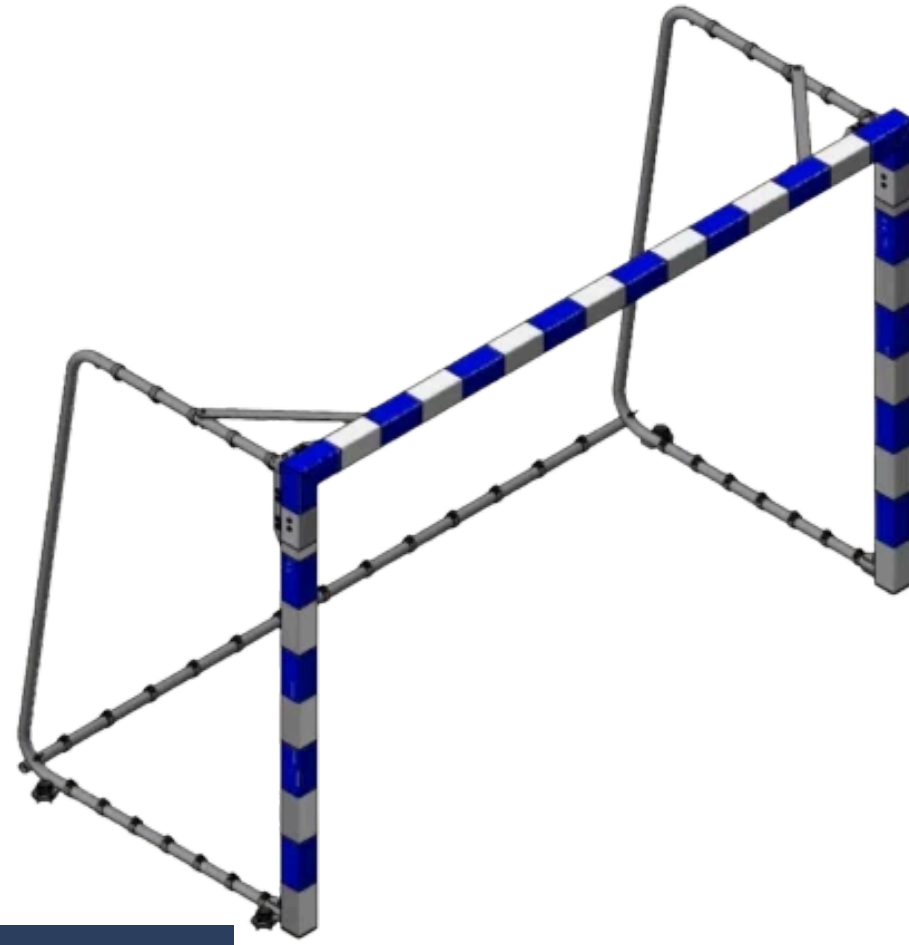
SU-50064 MINI HANDBALL GOAL USING SIZE: 2.4×1.6 M WEIGHT : 75KG
